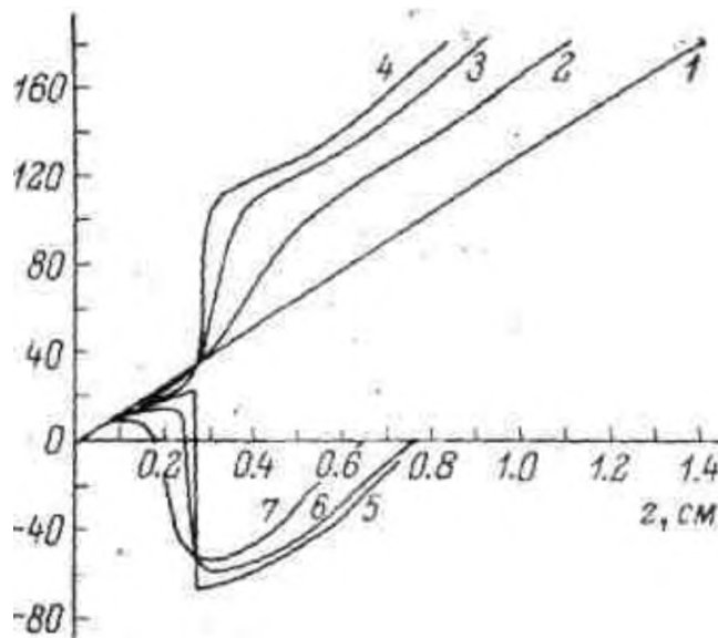
Рис. 3. Зависимость азимута \chi суммарного волнового поля в кристалле кварца от расстояния Z для малых углов, которому соответствует критическая ситуация (16), происходит за счет перемены местами большой и малой полуосей эллипса поляризации [3].
