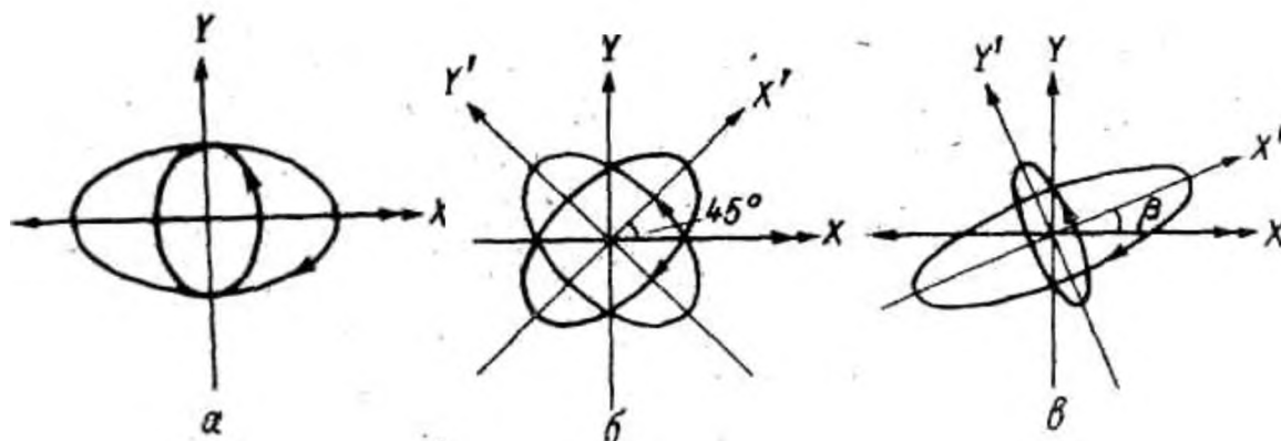
Рис. 1. Поперечные нормальные волны в кристалле кварца при поляризации падающей упругой волны, параллельной оси X , для трех случаев разориентации образца относительно оси Z . a — в плоскости YZ , b — при разориентации в произвольной плоскости ZX (в обоих случаях \nu = 1 ГГц, \theta = 1' ), c — при разориентации в произвольной плоскости.
