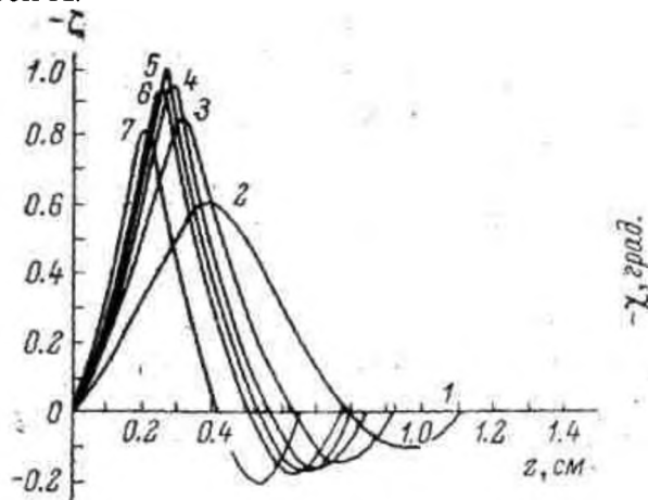
Рис. 2. Зависимость эллиптичности \xi = \text{tg}\delta суммарного волнового поля от расстояния Z в кристалле кварца при различных углах разориентации (мин). 1 - 0, 2 - 1.0, 3 - 1.5, 4 - 1.75, 5 - 1.88, 6 - 2.0, 7 - 2.5. Расчет по формуле (13), \gamma = 1.47 \cdot 10^4 дн/см.
