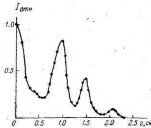
Рис. 5. Зависимость интенсивности рассеяния света на упругих волнах от расстояния Z в кристалле кварца. Измерения при частоте упругих волн 1.02 ГГц. Значение Z=0 соответствует первому максимуму интенсивности, считая от начала кристалла.
