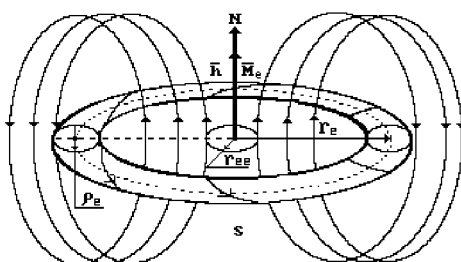
Рис. 1. схема теоретической модели электрона (показана лишь часть магнитных силовых линий).
