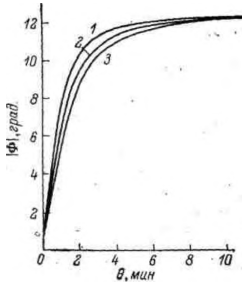
Рис. 4. Зависимость абсолютной величины угла рефракции для кварца от угла разориентации образца при различных частотах упругих волн \nu , ГГц: 1-1.02, 2-1.30, 3-1.55. Расчет по формуле (17) \gamma = 1.47 \cdot 10^4 дн/см
