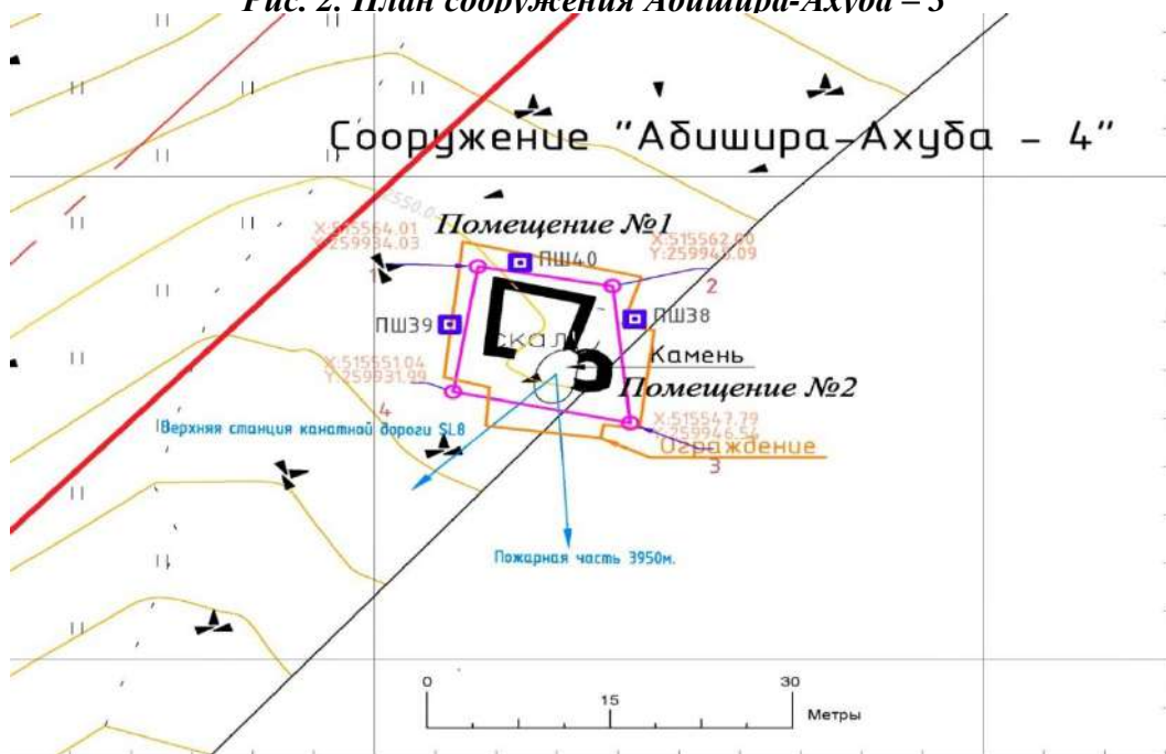
Рис. 3. План сооружения Абишира-Ахуба – 4
